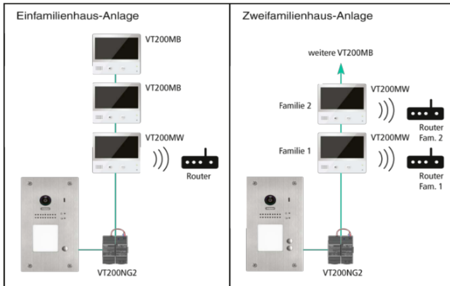
Abb. 3: VT200 bei Verwendung der Touch-Innenstation VT200MB
