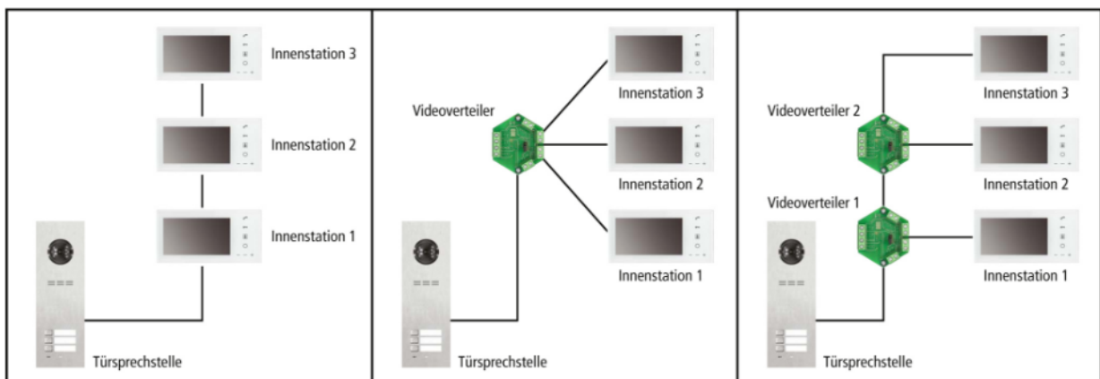
Abb. 1: Beispielhafte Verkabelungen VT100 (vereinfacht, nicht vollständig, nur zur Verdeutlichung der Videoverkabelung)
