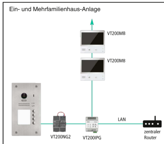
Abb. 4: Beispielhafte Verkabelungen VT200
