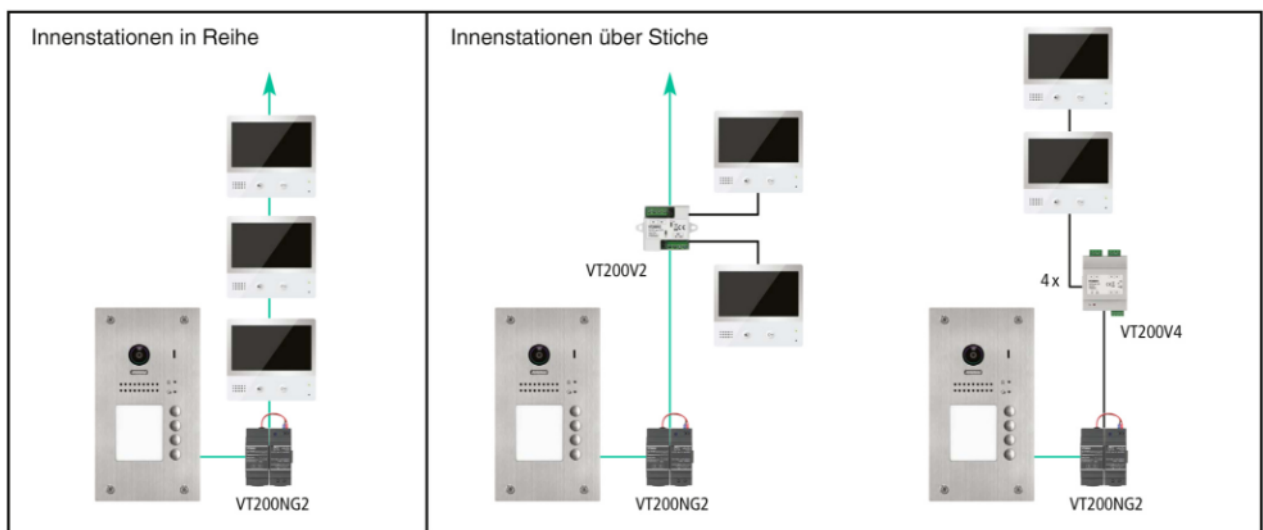
Abb. 4: Beispielhafte Verkabelungen VT200
